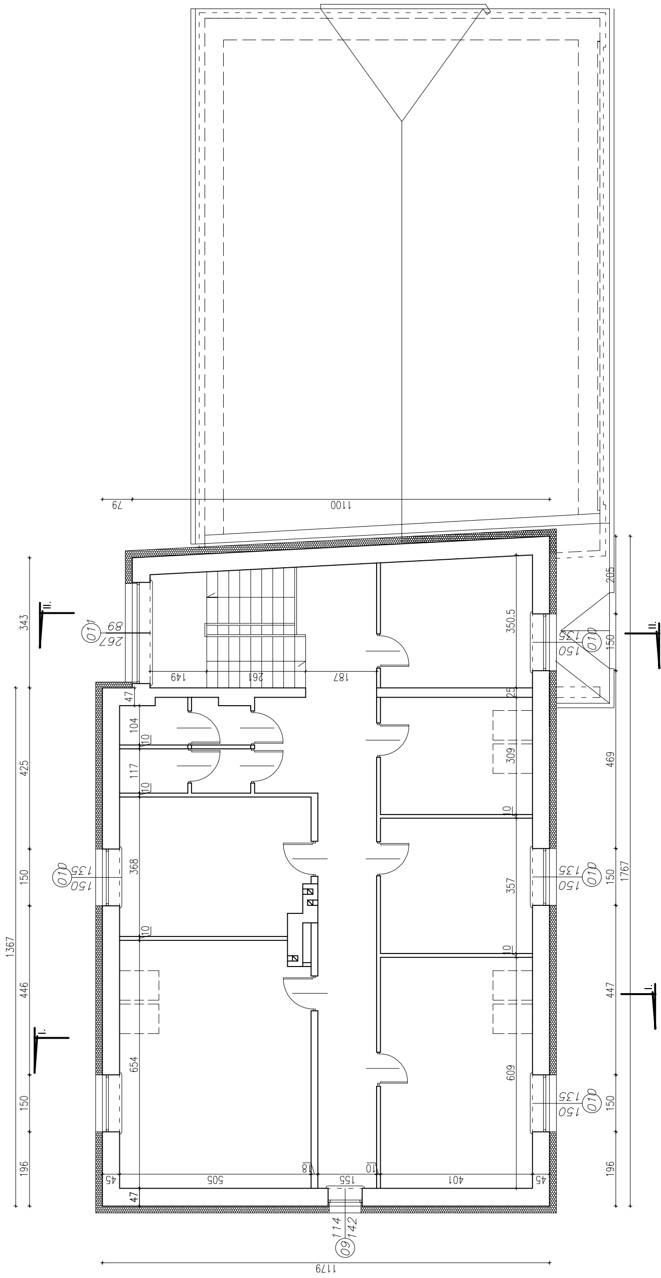
RZUT PODDASZA skala 1:100
